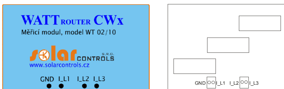
Obrázek 2: Popis svorek měřicích modulů WATTrouter CWx (pohledy shora) pro modely CWx a CWx SSR (vlevo) a CWx MAX (vpravo).
